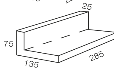
MTL75 ulkokulma 285/135x75 MTL75 yläkulma 285/135x75
