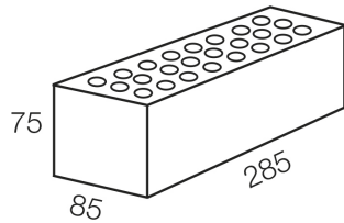
MRT75 285x85x75 mm
