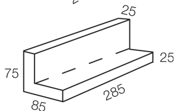
MTL75 ulkokulma 285/85x75 MTL75 yläkulma 285x85/75
